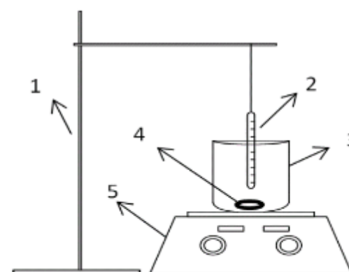
Gambar 1. Rangkaian Alat Isolasi Cangkang Bekicot menjadi kitosan
