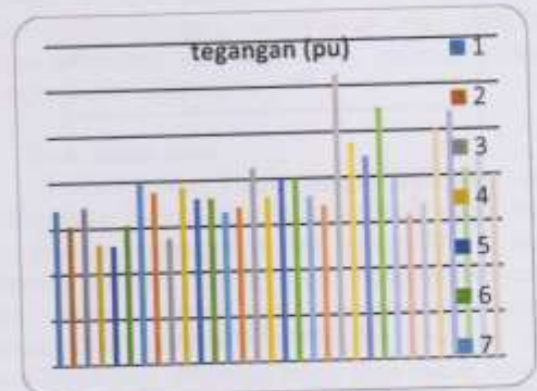
Gbr. 5 Profile tegangan (pu) pada setiap bus dengan kompensasi kapasitor 80MVar pada bus No.21.
