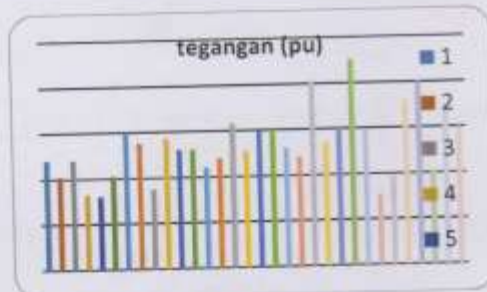
Gbr. 3 Profile tegangan (pu) pada setiap bus tanpa kapasitor
