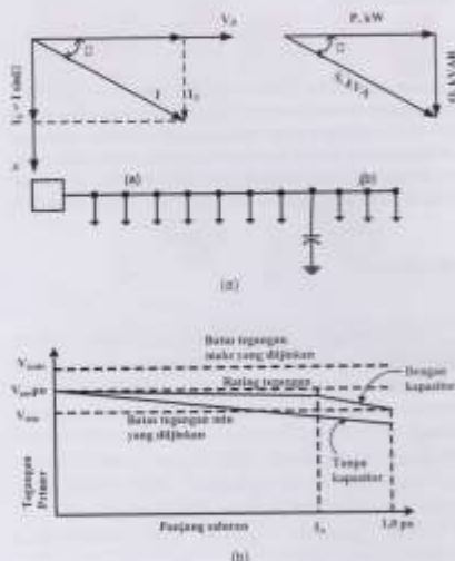
Gbr. 1 Hubungan antara daya aktif dan reaktif pada saluran
