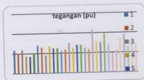
Gbr. 4 Profile tegangan (pu) pada setiap bus dengan kompensasi kapasitor 40MVar pada bus No.21.
