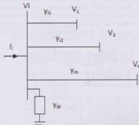
Gbr. 2 Suatu Sistem bus
