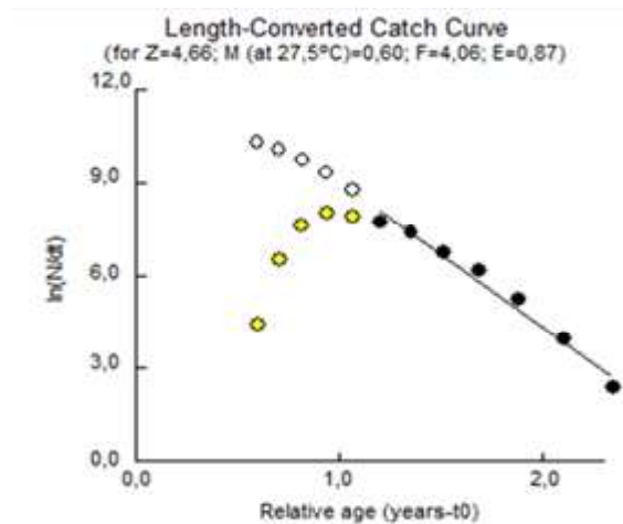
Gambar 5. Kurva hasil tangkapan yang mengkonversi panjang ikan beloso secara keseluruhan. Figure 5. The catch curve that converts the overall length of beloso fish.
