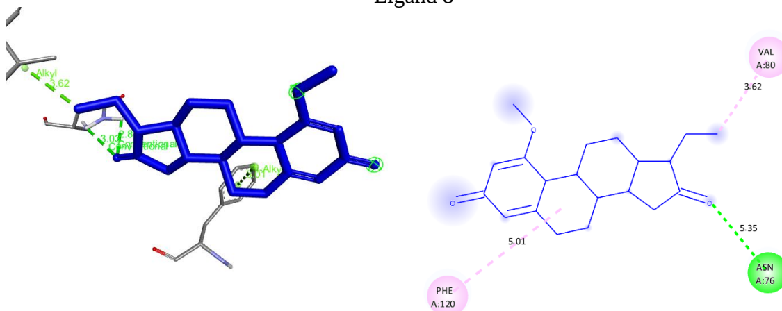
Ligand 8
