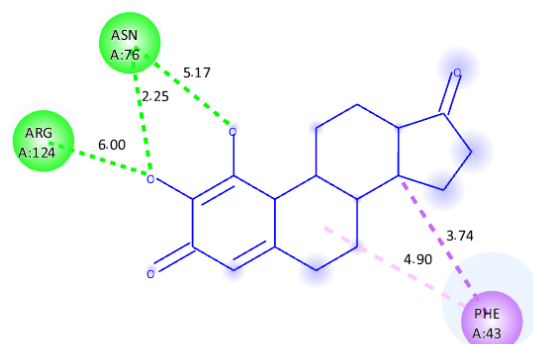
Ligand 4
