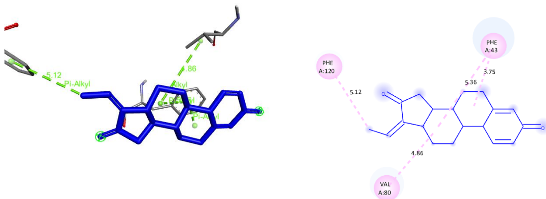
Ligand 6
