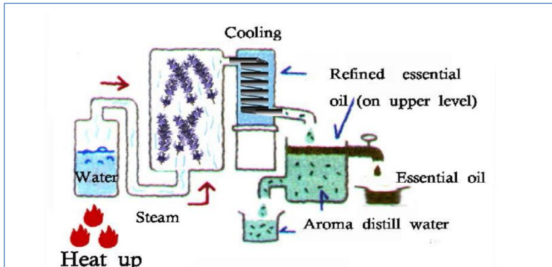
Gambar .alat destilasi uap air dalam pembuatan minyak menguap/esensial oil.
