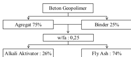
Gambar 1. Skenario struktur bahan
