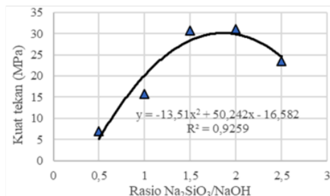
Gambar 4. Hubungan kuat tekan beton versus rasio Na 2 SiO 3 /NaOH umur 28 hari
