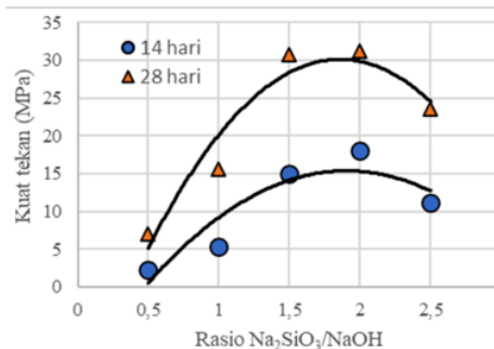
Gambar 2. Grafik hubungan antara kuat tekan beton versus rasio \text{Na}_2\text{SiO}_3/\text{NaOH}
