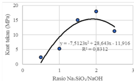
Gambar 3. Hubungan kuat tekan beton versus rasio Na 2 SiO 3 /NaOH umur 14 hari
