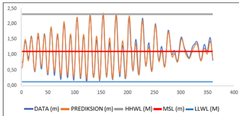
Fig 3: Tidal Charts
