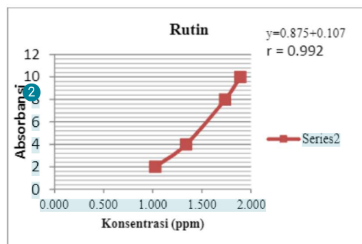
Gambar 2. Kurva kalibrasi rutin pada panjang gelombang 415 nm
