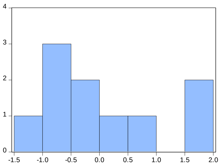
Gambar 2: Uji Normalitas
