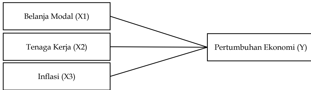
Gambar 1: Kerangka Konseptual
