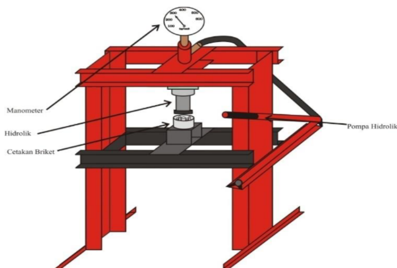
Gambar 1. Mesin press
