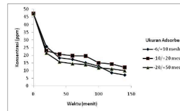
Gambar 4 Penurunan Konsentrasi Dodecyl Benzene Sulfonate (DBS) setiap selang waktu 20 menit
