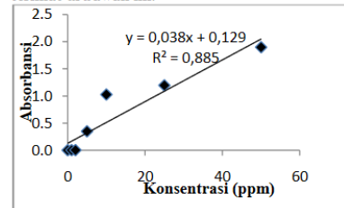
Gambar 2. Kurva Kalibrasi DBS
