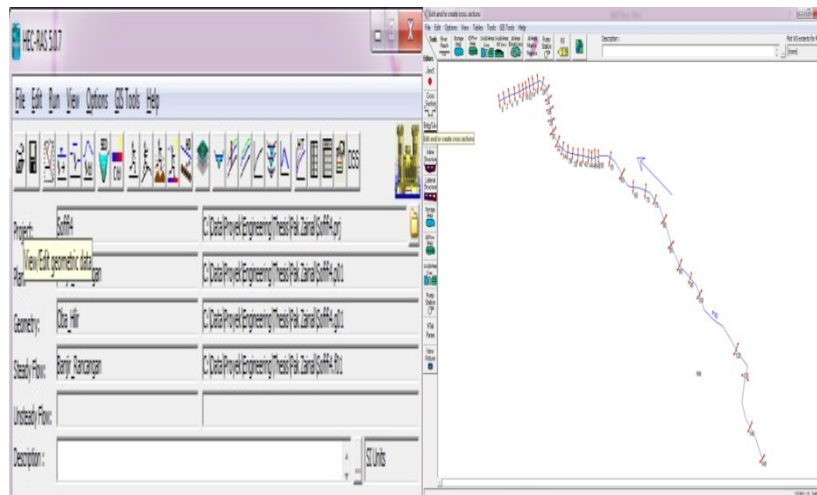
Gambar 4. Gambar perintah view/ edit geometric data dan Pembuatan Potongan Melintang (sumber: HEC-RAS 5.0.7 )
