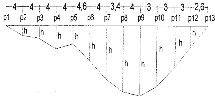
Gambar 4. Penampang melintang Bagian Tengah Sungai Maros
