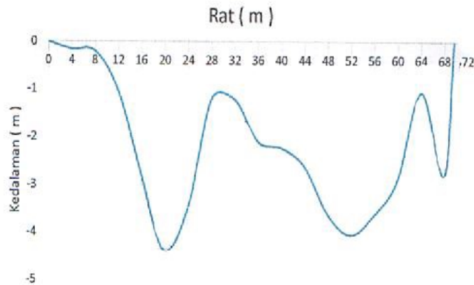
Gambar 3. Grafik Hubungan Antara Jarak Titik dan kedalaman Penampang Hilir sungai Maros
