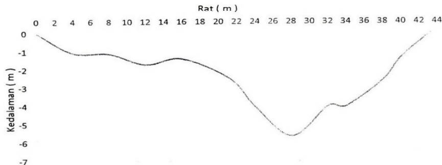
Gambar 2. Grafik hubungan antara rat dan kedalaman penampang tengah Sungai Maros
