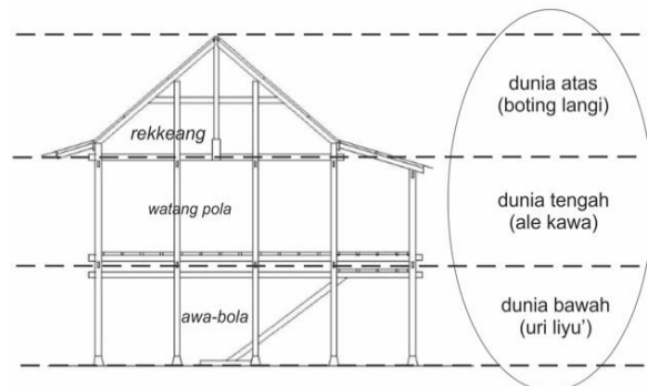
Gambar 2 Ale Bola/Watang pola pada Potongan Rumah Bugis
